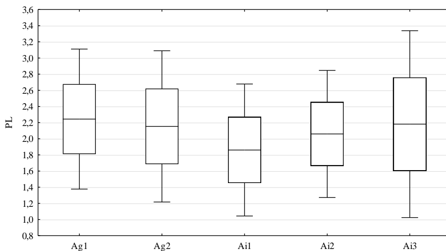
Slika19. Osnovni statistički parametri za dužinu peteljke (PL) prikazani Box & Whiskers dijagramima. Box : aritmetička sredina \pm standardna devijacija, whiskers : aritmetička sredina \pm 2 \times standardne devijacije.
