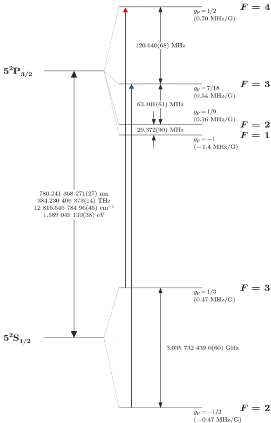
Slika 2.5: Hiperfini energijski nivoi ^{85}\text{Rb} . Crvenom strelicom označen je prijelaz lasera za hlađenje, a plavom lasera za naseljavanje. Preuzeto iz [11].
