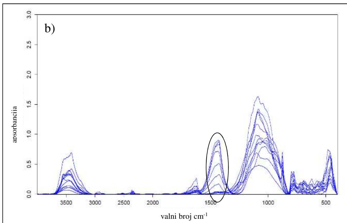
Slike 42 i 43. FT-IR spektri uzoraka iz kopnenih (a) i morskih nalazišta (b)
