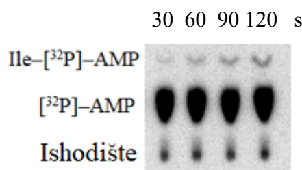
Slika 4.24. Reprezentativni kromatogram Ile- ^{32}\text{P} -AMP i [ ^{32}\text{P} ]-AMP razdvojenih tankoslojnom kromatografijom. Analizirani su alikvoti reakcije u vremenskim intervalima kako slijedi s lijeva na desno: 30, 60, 90, 120 s.
