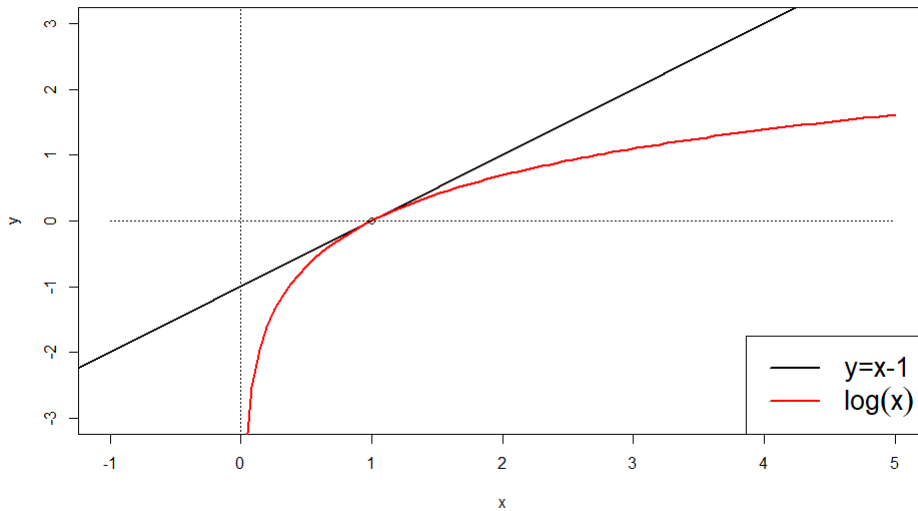
Slika 1.4: Grafovi funkcija y = x - 1 i y = \log(x)
