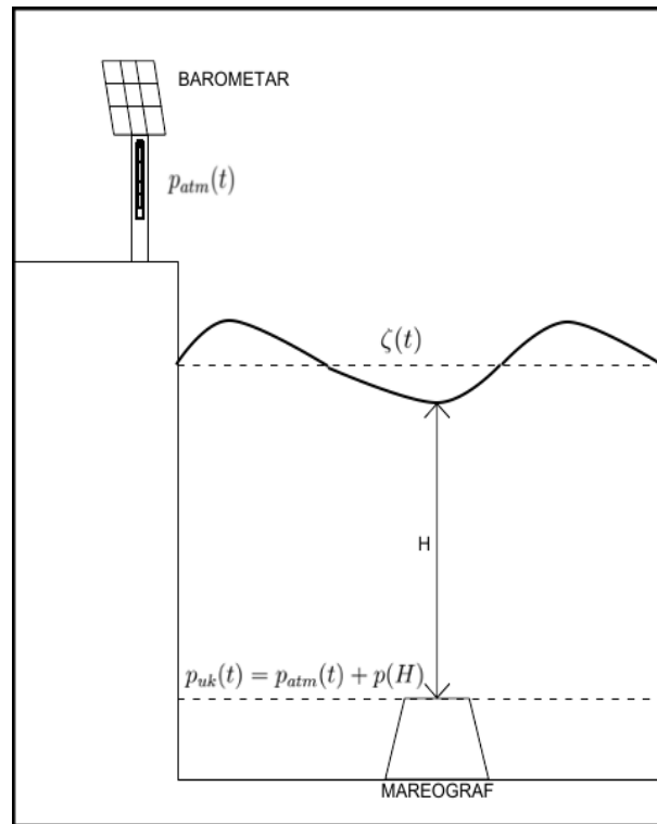
Slika 3.1. Skica mjernog postava. \zeta je denivelacija mora računata po jednadžbi 2.9, p(H) je tlak koji stupac morske vode visine H vrši na mjerni uređaj, p_{atm} je prizemni atmosferski tlak u obližnjoj točki, a p_{uk} je tlak koji je mjerio mareograf.
