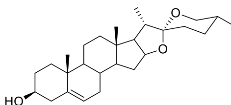
Slika 6. Struktura diozgenina.
