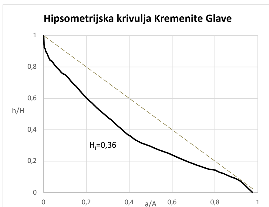
Slika 39. Hipsometrijska krivulja drenažnog bazena Kremenite Glave
