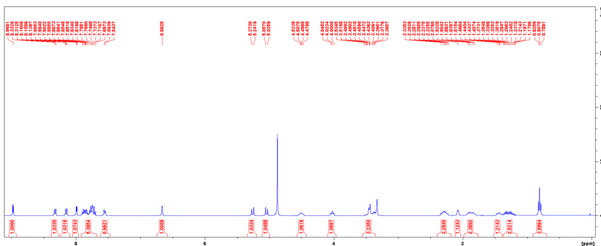
Slika D16. ^1\text{H} NMR spektar spoja 16
