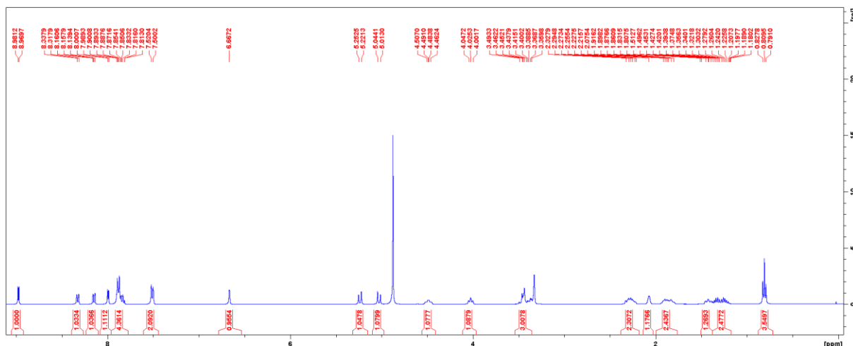
Slika D17. 1 H NMR spektar spoja 17
