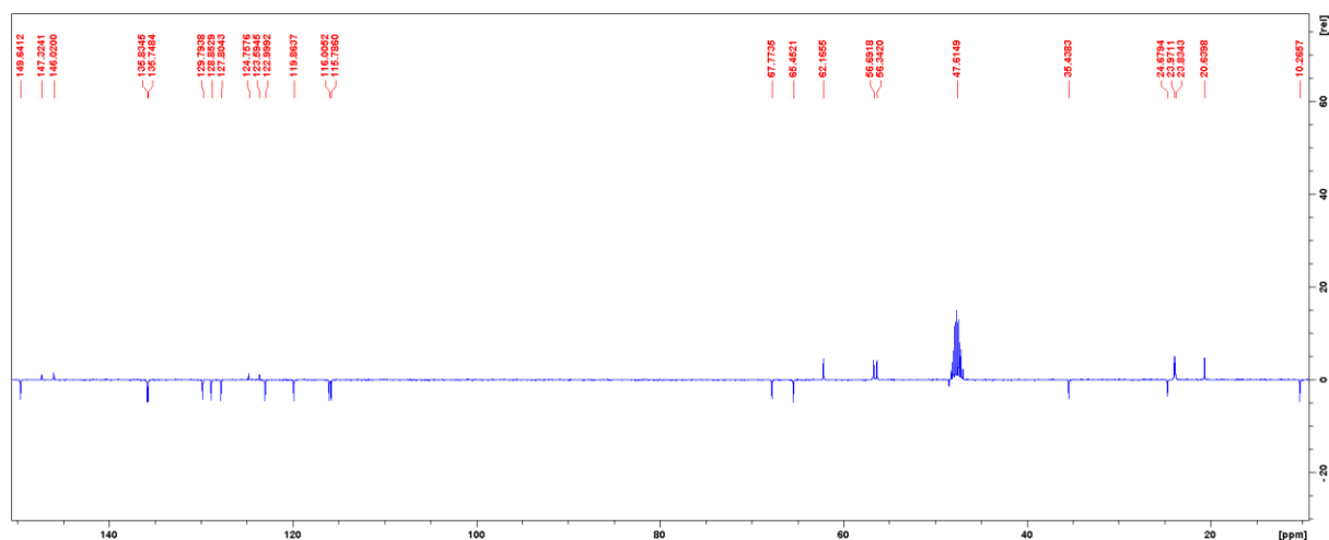
Slika D23. ^{13}\text{C} NMR spektar spoja 5
