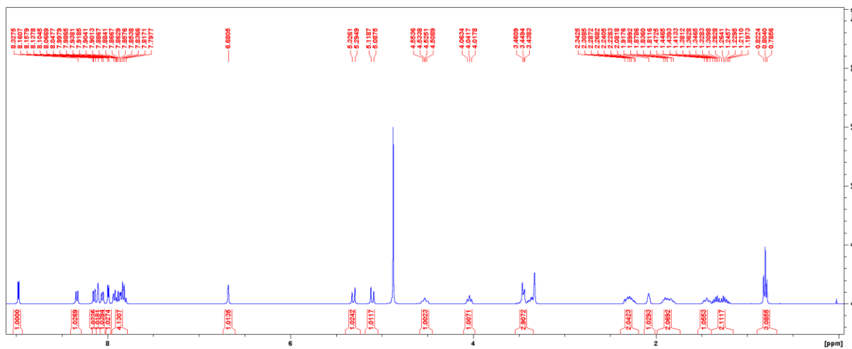
Slika D15. ^1\text{H} NMR spektar spoja 15
