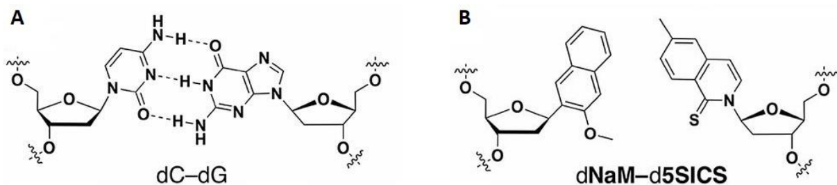
Slika 10. Prikaz dC-dG i dNaM-d5SICS baznih parova. (A) Kemijska struktura parova baza dC-dG i (B) dNaM-d5SICS.
