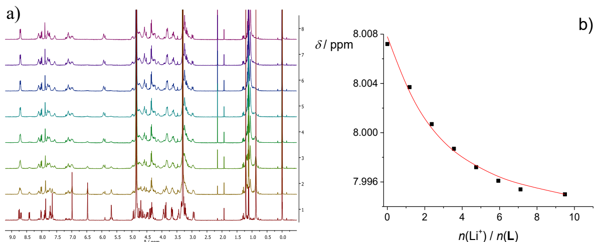
Slika 7. a) Titracija ^1\text{H} NMR spoja L ( c = 1,42 \times 10^{-3} \text{ mol dm}^{-3} ) s litijevim perkloratom ( c = 1,51 \times 10^{-1} \text{ mol dm}^{-3} ) u MeOD pri 25 \text{ }^\circ\text{C} . b) Ovisnost kemijskog pomaka protona na 8,01 ppm o omjeru množina dodanog \text{LiClO}_4 i spoja L .
