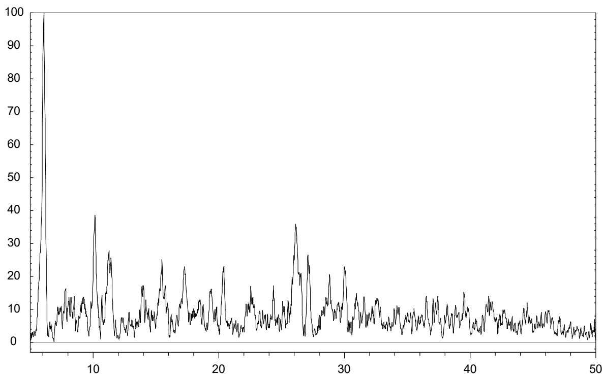
Slika D41. Difraktogram prahe uzorka O1-a dobivenog metodom D.
