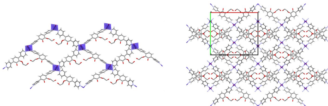
Slika 5. Jedan sloj (lijevo) i pakiranje koordinacijskog polimera [\{Co(L)_2(H_2O)_2\}(NO_3)_2 \cdot 1,5H_2O\}_n duž osi c (desno). Solvatirane molekule vode i nitratni anioni su radi jednostavnosti prikaza izostavljeni.
