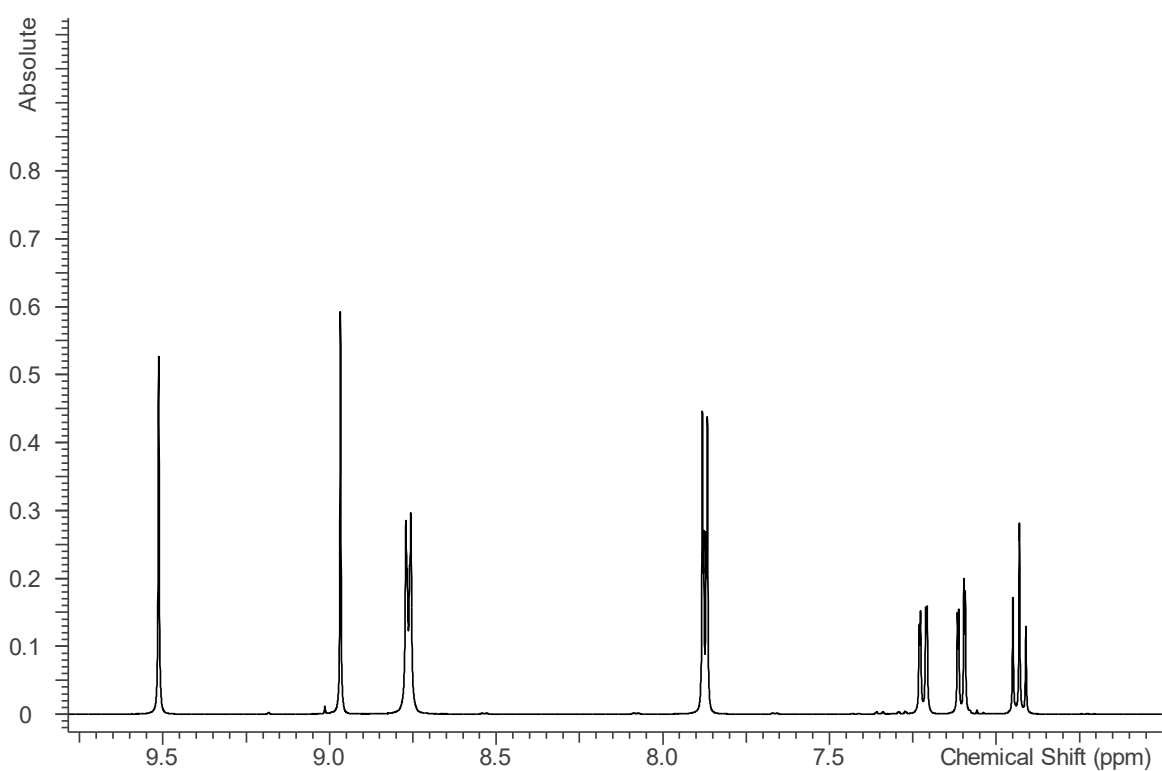
Slika D21. Uvećani prikaz 1 H spektra 3 · acetone
