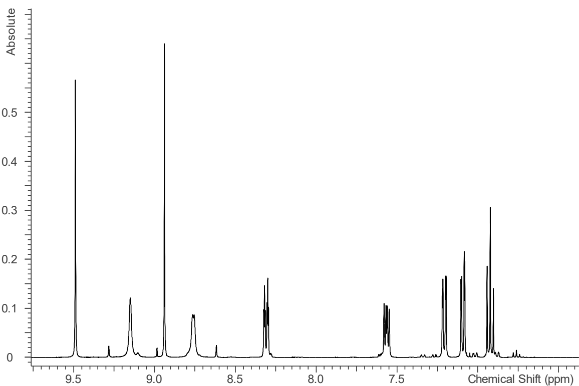
Slika D29. Uvećani prikaz 1 H spektra 4 · acetone
