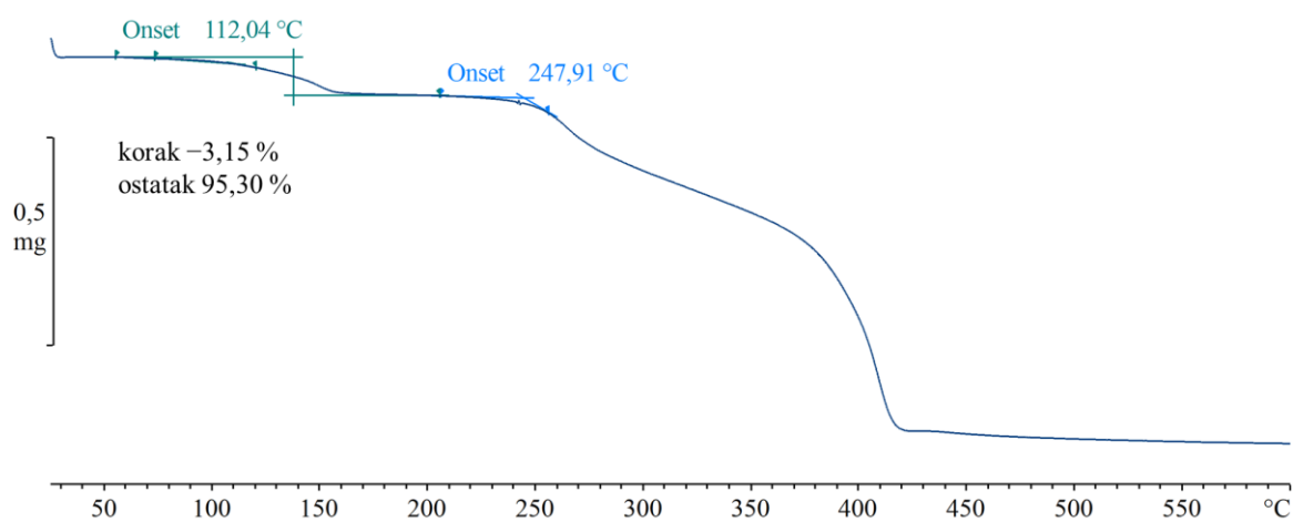
Slika 43. Termogram raspada O2 . Pad mase na početku mjerenja (ispod 50^{\circ}\text{C} ) pripisan je nedovoljnoj posušenosti uzorka zbog kojeg je zbroj postotaka pada mase u prvom koraku i ostatka manji od 100 %.
