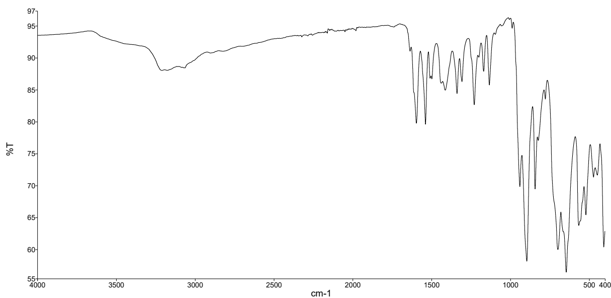
Slika D14. IR spektar uzorka spoja O1 · 4MeCN · 2H 2 O nakon snimanja difraktograma prahe. Može se uočiti kako usitnjavanjem dolazi do izlaska acetonitrila i vode.
