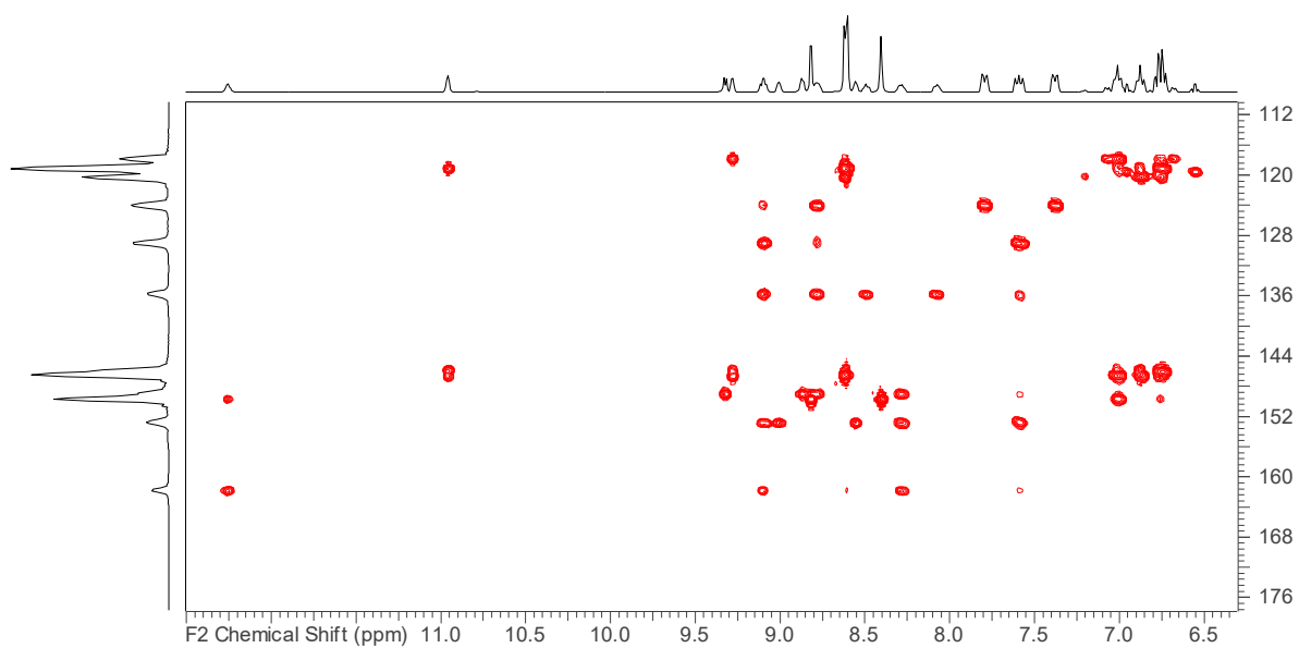
Slika D28. Uvećani prikaz HMBC spektra H 2 L 4
