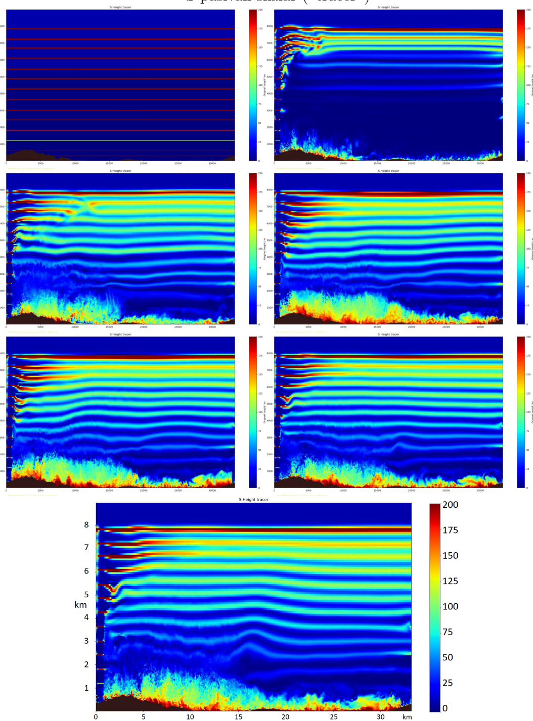
Slika 24 YZ presjek sedam izdvojenih trenutaka simulacije nakon 0 s, 820 s, 1640 s, 4510 s, 9050 s, 13600 s, 18000 s (s lijeva na desno prema niže). S pasivan skalar prikazan je bojom, dok je zacrnjeno područje ispod površine zemlje. Sinoptički vjetar puše u smjeru osi z na grafu (prema čitatelju).
