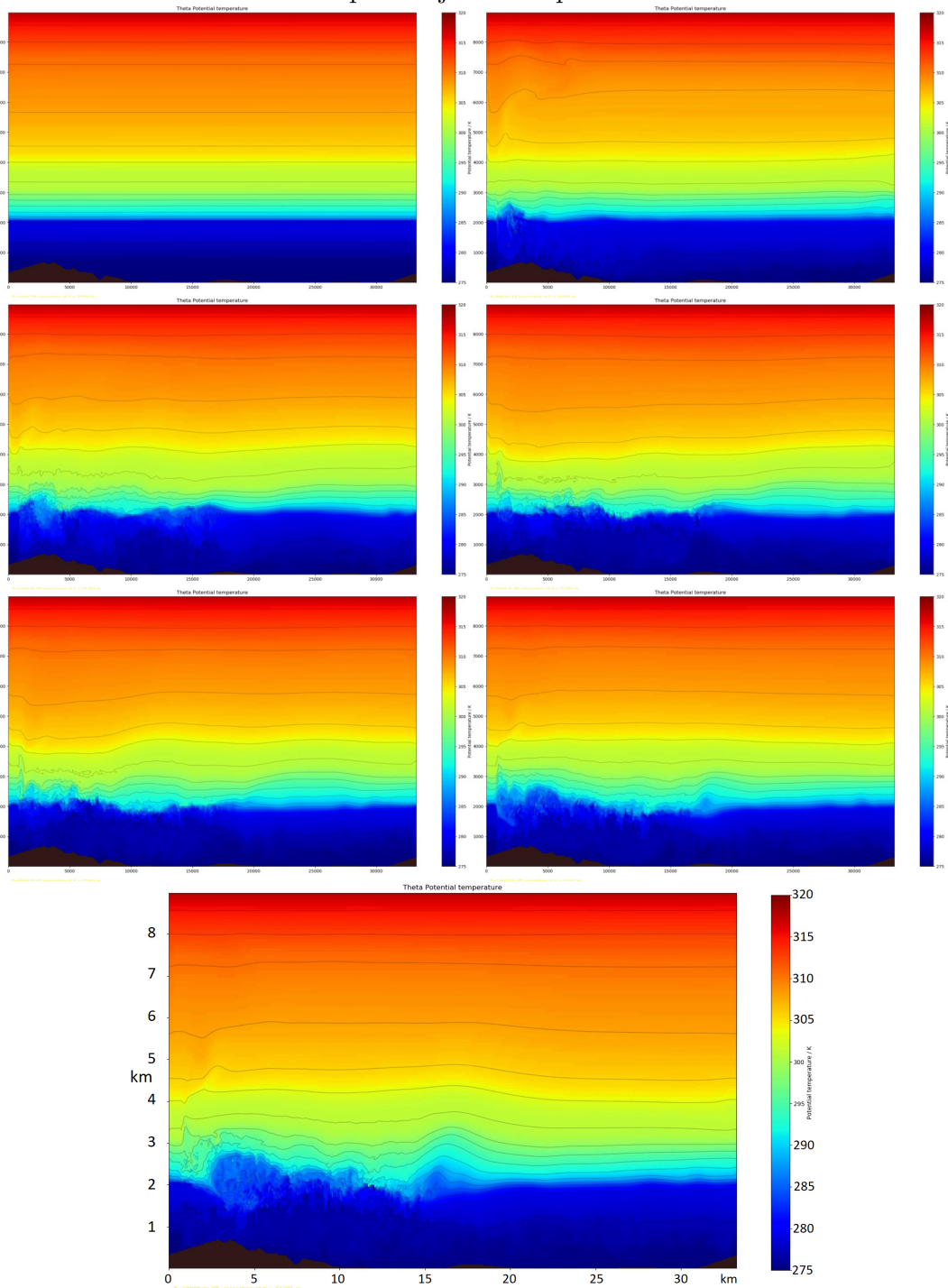
Slika 20 YZ presjek sedam izdvojenih trenutaka simulacije nakon 0 s, 820 s, 1640 s, 4510 s, 9050 s, 13600 s, 18000 s (s lijeva na desno prema niže). \theta u K prikazana je bojom, dok je zacrnjeno područje ispod površine zemlje. Sinoptički vjetar puše u smjeru osi z na grafu (prema čitatelju).
