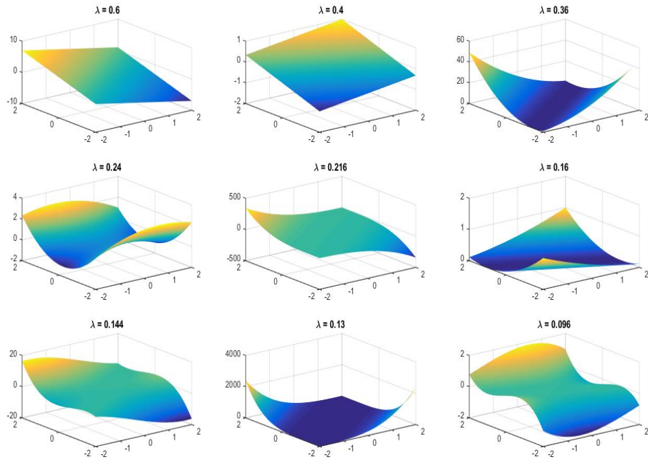
Slika 3.1: Prvih devet svojstvenih vrijednosti (osim trivijalne 1) i pripadajuće svojstvene funkcije Koopmanovog operatora dobivene aproksimacijom polinomima stupnja manjeg ili jednagog 5.
