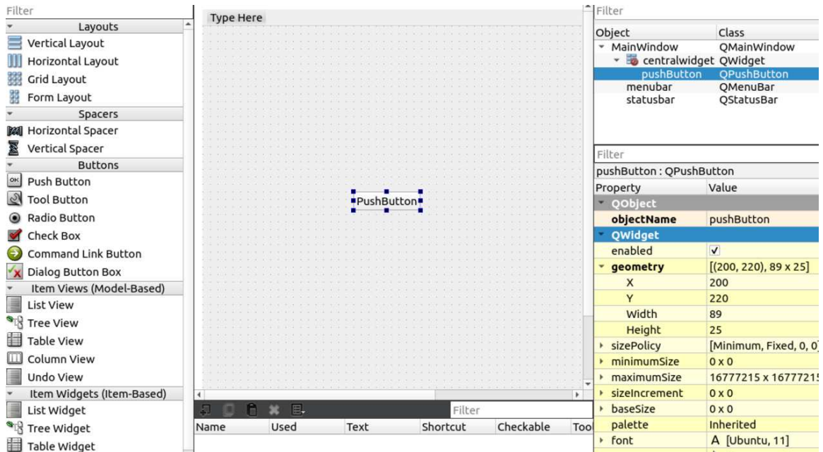
Slika 1.5: Qt Designer
