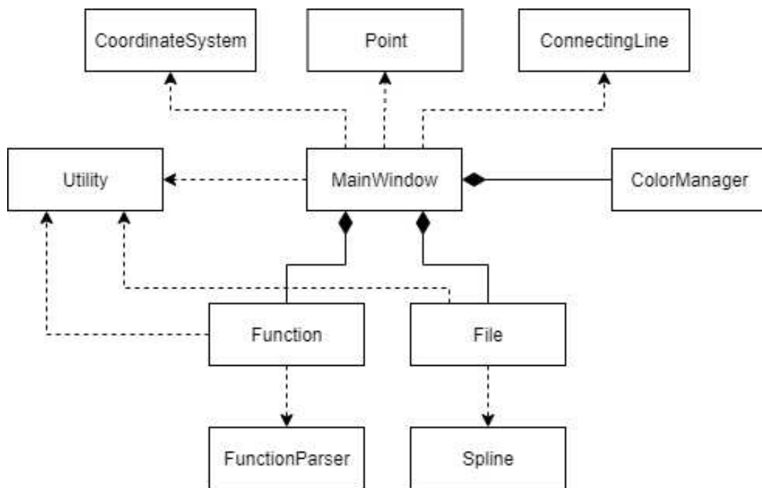
Slika 2.17: Struktura aplikacije
