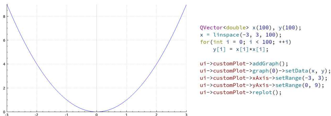
Slika 2.1: Primjer QCustomPlot grafa s pripadajućim kodom
