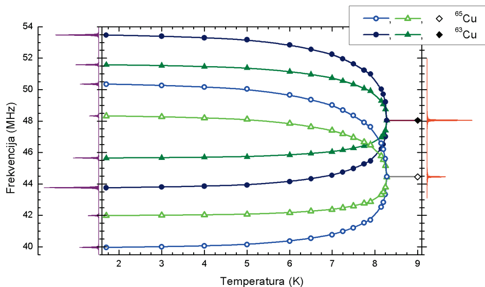
Slika 3.15: NQR signal bakra u nultom magnetskom polju. Cijepanje jedne linije na četiri nastaje zbog razvoja statičkog magnetskog momenta u antiferomagnetskoj fazi. Razmak linija proporcionalan je s unutrašnjim magnetskim poljem na mjestu jezgre Cu1.
