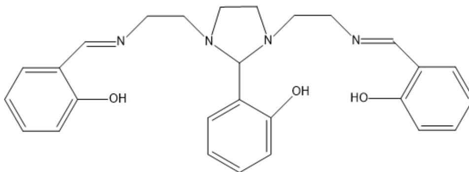
Slika 9. Molekulska struktura H 3 L
