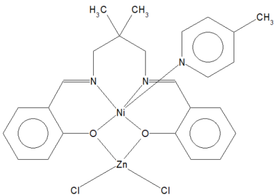
Slika 6. Kompleks (2) NiLDM · ZnCl 2 · 4-pikolin
