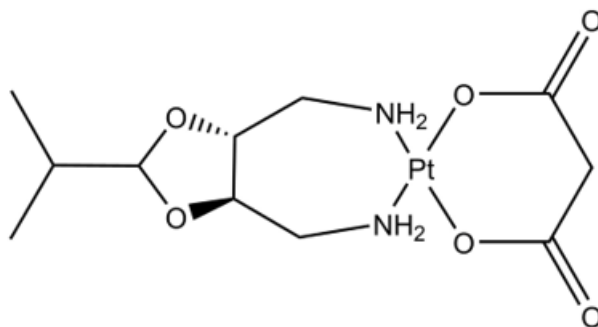
Slika 11. Struktura heptaplatina.
