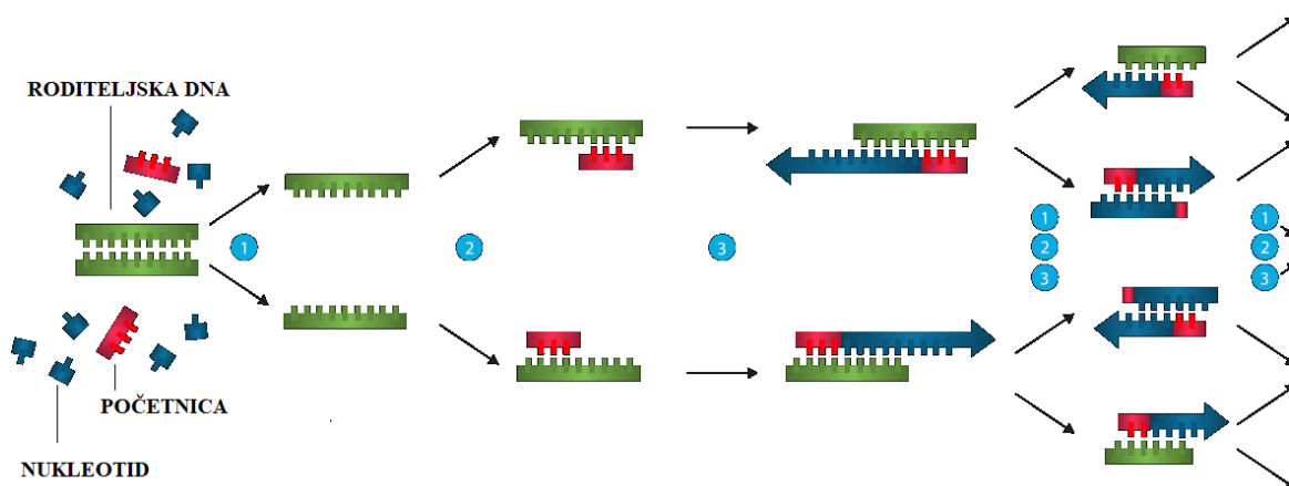
Slika 9. Faze PCR metode – prema 21
