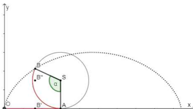
Slika 1.3: Cikloida
