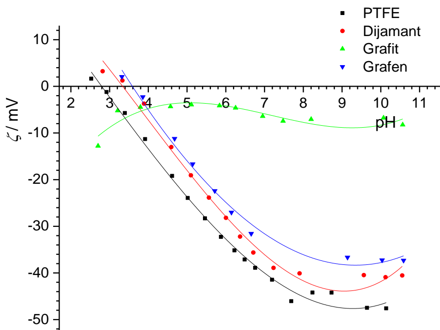
Slika 5.17. Vrijednosti elektrokinetičkog potencijala PTFE, dijamanta, grafita i grafena tijekom potenciometrijske titracije vodene otopine NaCl ( I_c = 2 \text{ mmol dm}^{-3} ). \theta = 40 \text{ }^\circ\text{C} .
