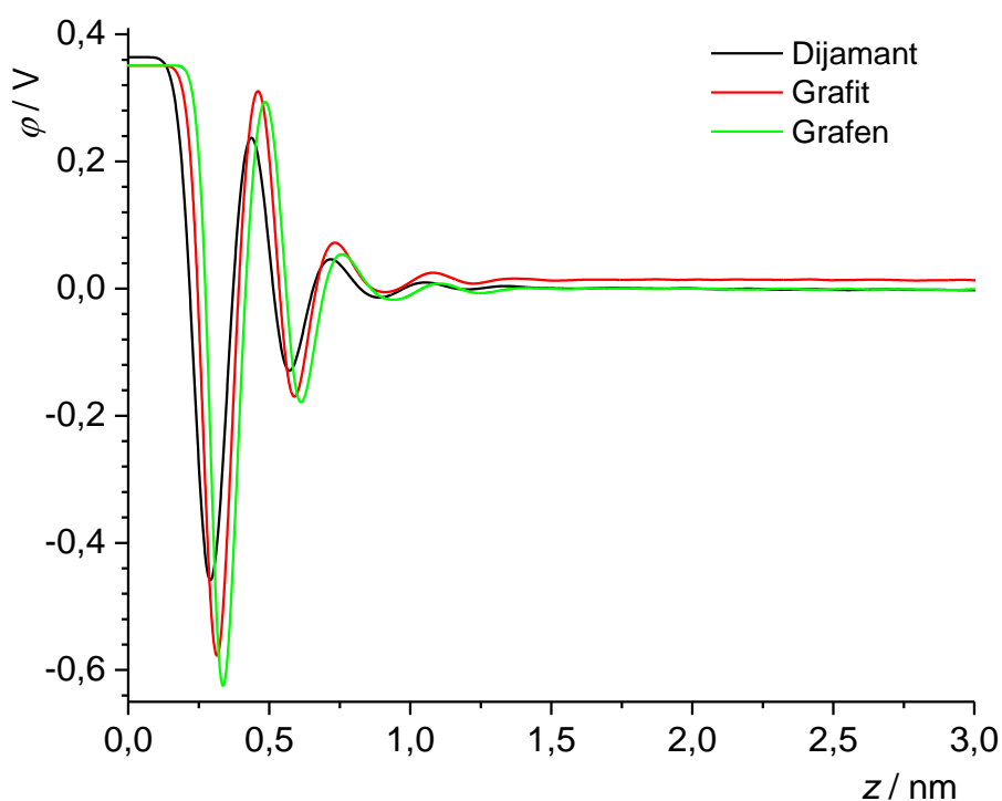
Slika 5.64. Potencijal sustava za međupovršinu dijamant, grafit, grafen / vodena otopina NaCl.
