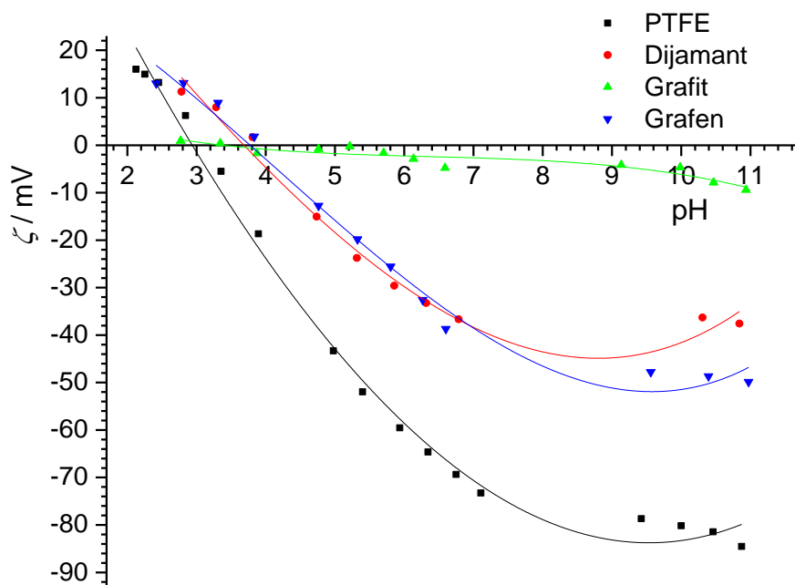
Slika 5.16. Vrijednosti elektrokinetičkog potencijala PTFE, dijamanta, grafita i grafena tijekom potenciometrijske titracije vodene otopine NaCl ( I_c = 2 \text{ mmol dm}^{-3} ). \theta = 25 \text{ }^\circ\text{C} .
