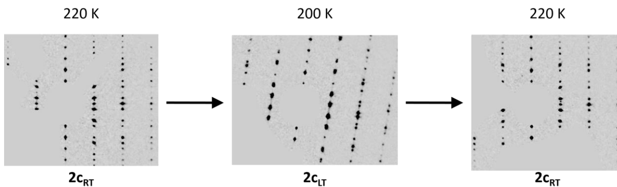
Slika D23. Precesijske slike polimorfa spoja 2c oko osi h0l . U polimorfu 2c LT mogu se uočiti udvostručeni difrakcijski maksimumi.
