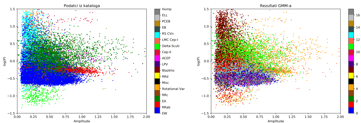
Slika 5.10: Usporedba klasifikacija promjenjivih zvijezda iz kataloga i klasifikacija prema GMM algoritmu preko amplituda - logaritama perioda grafa za 18 komponenti.
