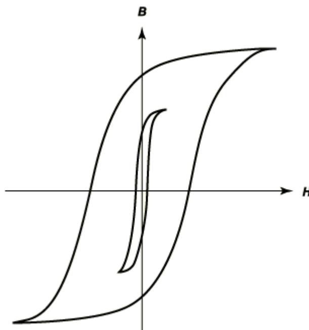
Slika 1.3: Krivulja histereze mekog i tvrdog magnetskog materijala [11].
