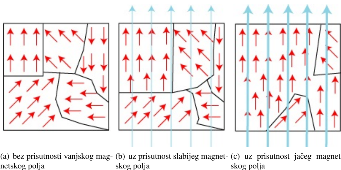
Slika 1.1: Weissove domene [9].
