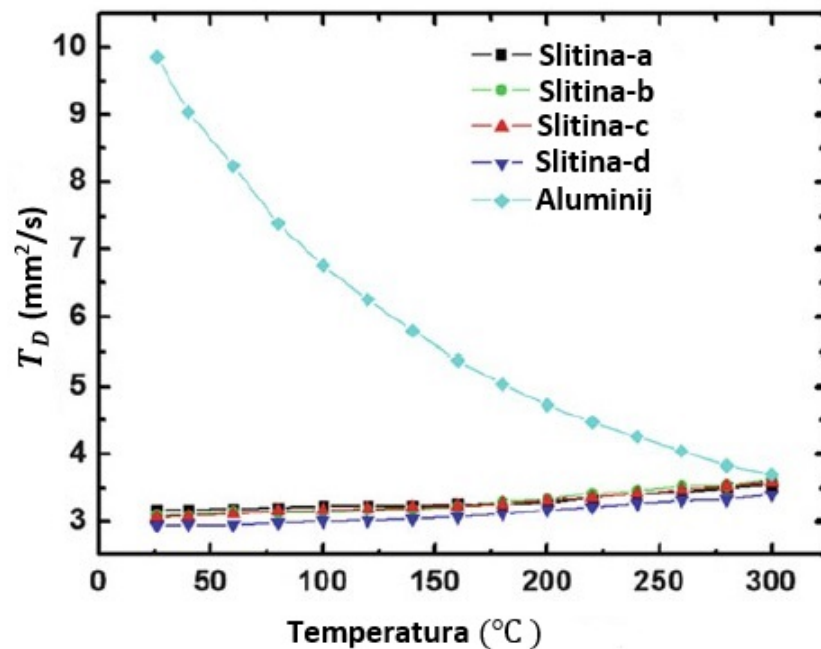
Slika 8.1: Toplinska difuzivnost kao funkcija temperature za neke viskoentropijske slitine i aluminij [13].
