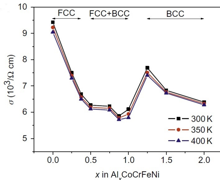
Slika 6.4: Električna vodljivost \text{Al}_x\text{CoCrFeNi} slitine u ovisnosti o x(uduo aluminija) [5].
