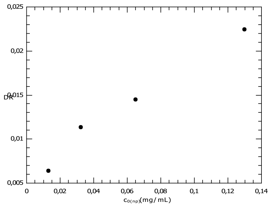
Slika 35. Stopa degradacije po masenoj koncentraciji nanočestica za RB
