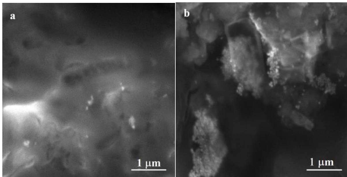
Slika 60. SEM mikrografija uzoraka koji prikazuju nanočestice srebra promjera 60 nm (Ag60 NC, 5 \mu\text{g mL}^{-1} s dodatkom Tweena 80 (1 \text{mg mL}^{-1} ) u filtriranoj morskoj vodi saliniteta 15 u prisutnosti: a) modelnog sedimenta, MMT-a i b) prirodnog sedimenta iz Linskog kanala, NS nakon 10 dana.
