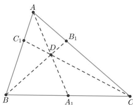
Slika 1.1: Cevin teorem
