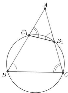
Slika 1.11: Antiparalela
