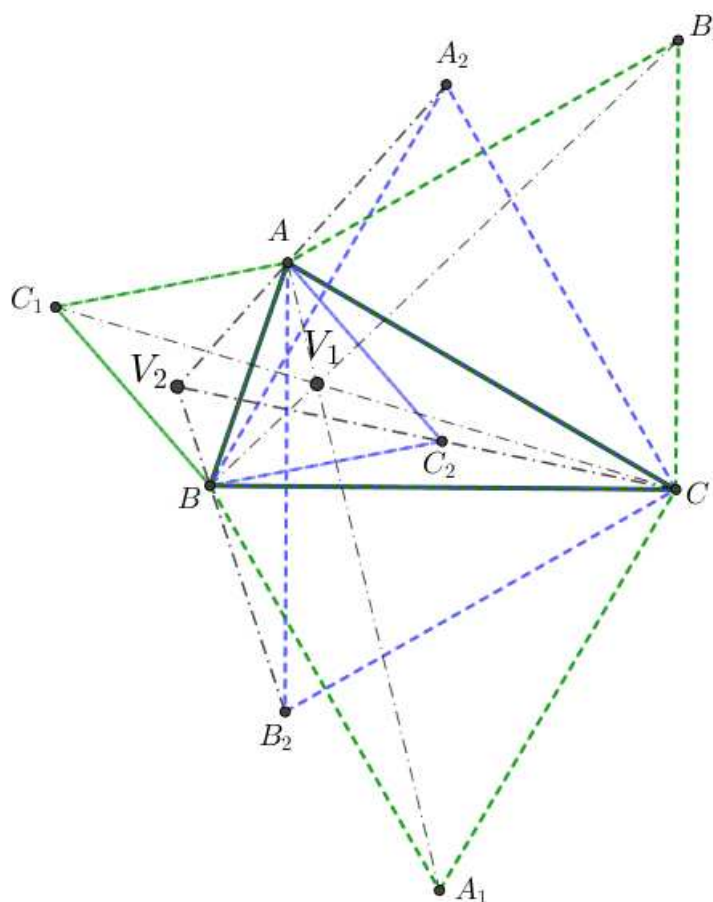
Slika 1.10: Izogonični centri
