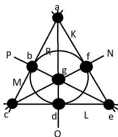
Slika 5: Fanova ravnina
