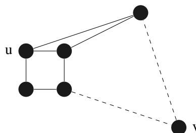
Slika 3.9: Graf G_2
