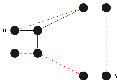
Slika 3.10: Bridno disjunktne (u, v) -putovi
