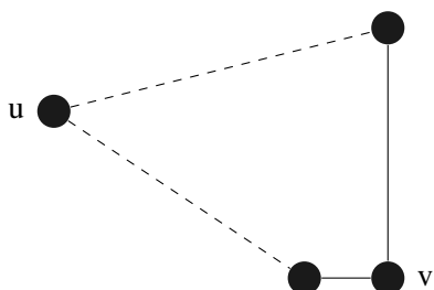
Slika 3.8: Graf G_1
