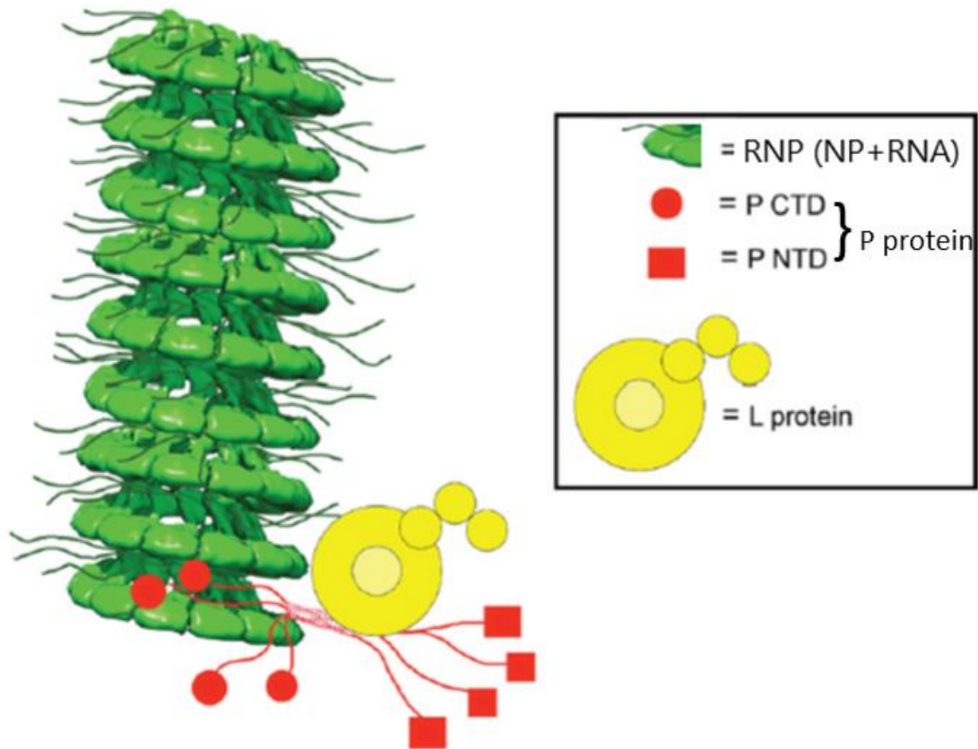
Slika 3. Model interakcija između nukleoproteina (NP), fosfoproteina (P) i velikog proteina (L). Virusna RNA-ovisna RNA polimeraza je kompleks proteina L i P. Protein NP s genomskom RNA formira ribonukleoprotein (RNP). Gola genomaska RNA ne može se replicirati ni transkribirati. Protein P odgovoran je za vezanje proteina L i NP interkacijama u P C-terminalnoj domeni (P CTD). Time se RNA-ovisna RNA polimeraza veže za RNP i počinje sintezu virusne RNA (preuzeto i prilagođeno iz (Cox i Plemper 2015).
