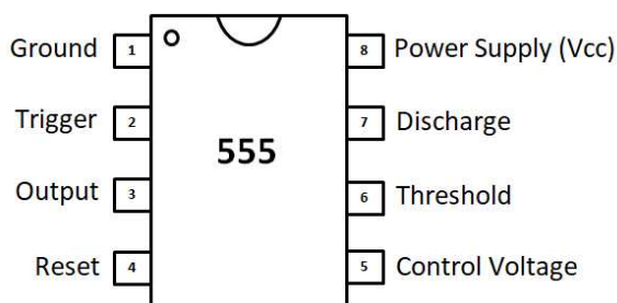
Tablica (1) – redosljed i funkcije pinova vremenskog sklopa 555.
