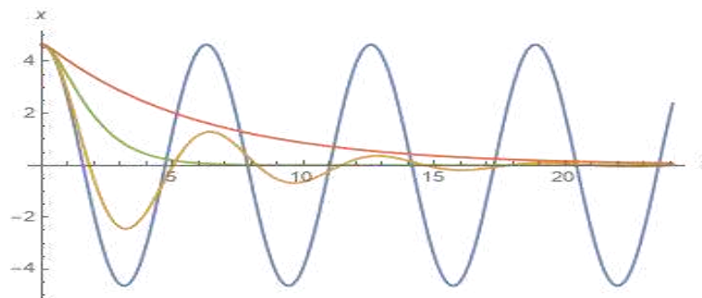
Slika (2) – primjer potkrično gušenog osciliranja (žuto), kritično gušenog osciliranja (crveno) i natkrično gušenog osciliranja (zeleno) u usporedbi sa slobodnim osciliranjem (plavo).
