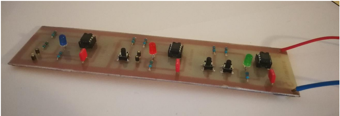
Slika (40) – završni proizvod – sklop dobiven upotrebom tiskane pločice.
