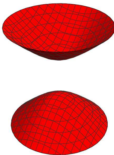
Slika 2.8: Dvoplošni hiperboloid
