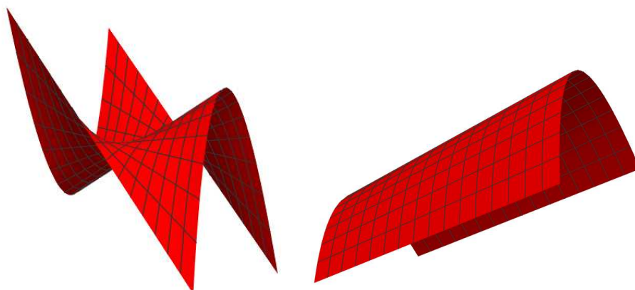
Slika 3.8: Parabolički konoid
