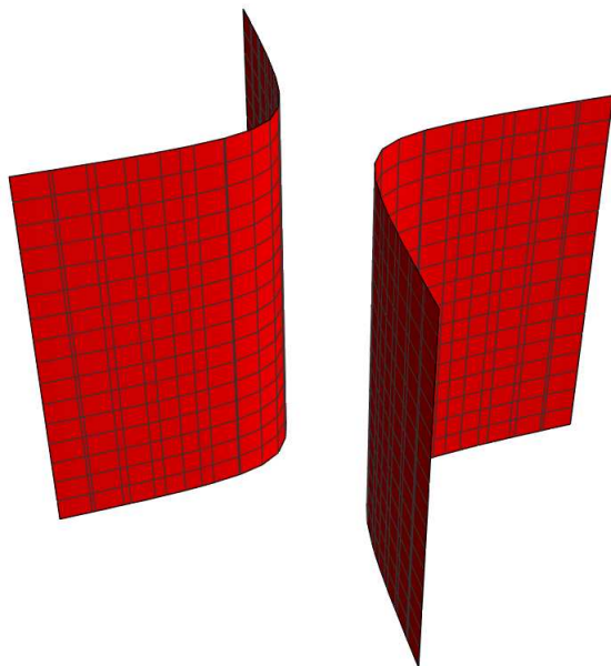
Slika 2.20: Hiperbolički valjak
