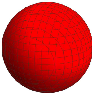
Slika 2.1: Sfera
