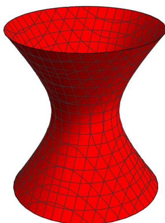
Slika 2.4: Jednoplošni hiperboloid
