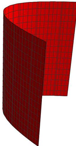
Slika 2.19: Parabolički valjak
