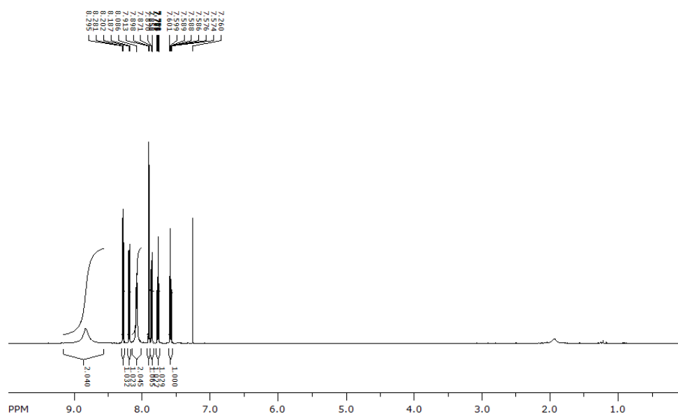
Slika D9. 1 H NMR spektar 2-(4-piridil)kinolina ( 3e )
