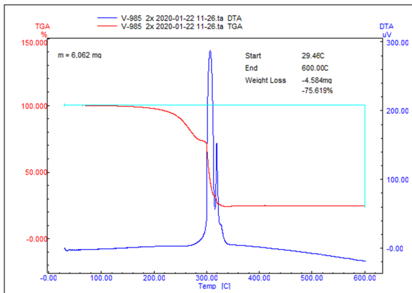
Slika 40. DTA i TGA krivulje spoja Cu(BDC)(DMF)
