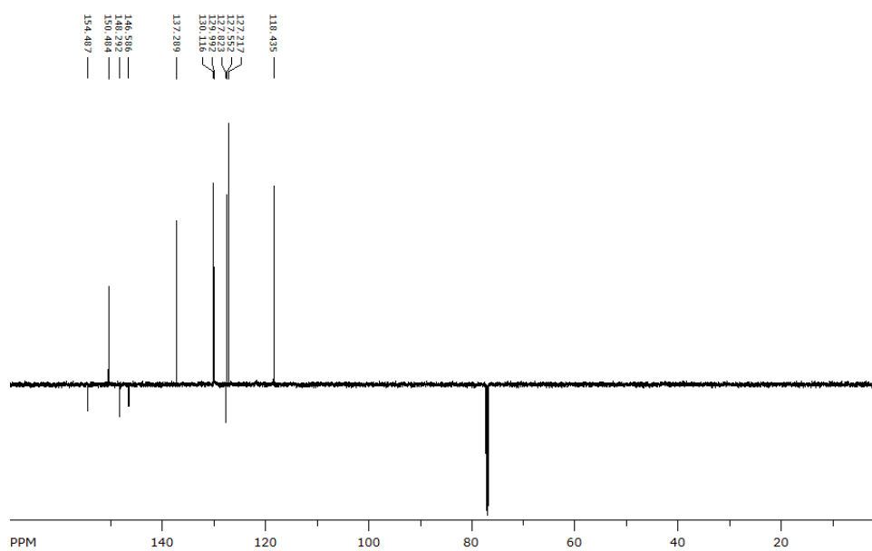
Slika D10. 13 C NMR spektar 2-(4-piridil)kinolina ( 3e )
