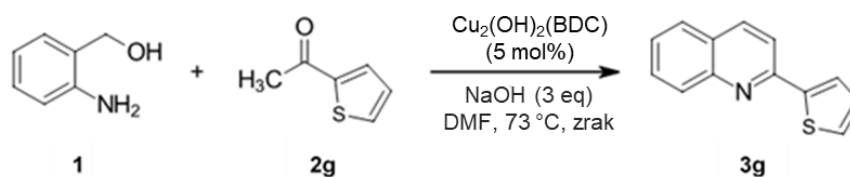
Slika 31. Reakcija 2-aminobenzilnog alkohola i 2-acetiltiofena za dobivanje 2-(2-tienil)kinolina
