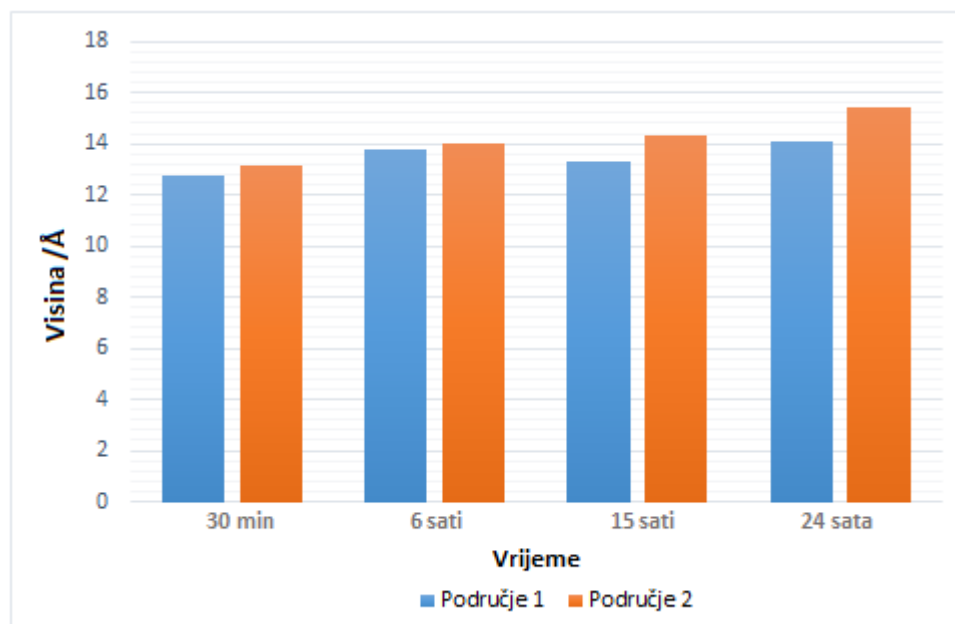
Slika 21. Prosječne visine „otoka“ molekularnih slojeva spoja 2c na površini zlata (111) određene analizom topografskih podataka prikupljenih AFM mikroskopijom za područja 1 i 2 pri različitim vremenima adsorpcije (30 min, 6 sati, 15 sati i 24 sata)
