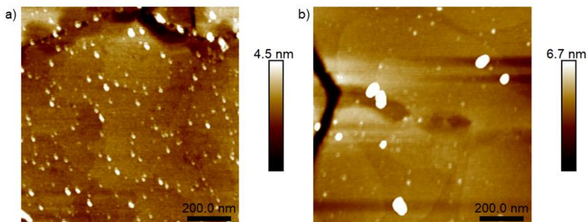
Slika D2. 1\ \mu\text{m} \times 1\ \mu\text{m} AFM slika a) molekularnog sloja nastalog uranjanjem supstrata zlata (111) u otopinu spoja 2c na 30 min i b) molekularnog sloja nastalog uranjanjem supstrata zlata (111) u otopinu spoja 2c na 15 sati.
