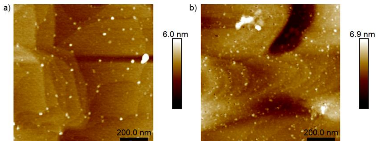
Slika D1. 1\ \mu\text{m} \times 1\ \mu\text{m} AFM slika a) molekularnog sloja nastalog uranjanjem supstrata zlata (111) u otopinu spoja 1c na 30 min i b) molekularnog sloja nastalog uranjanjem supstrata zlata (111) u otopinu spoja 1c na 15 sati.
