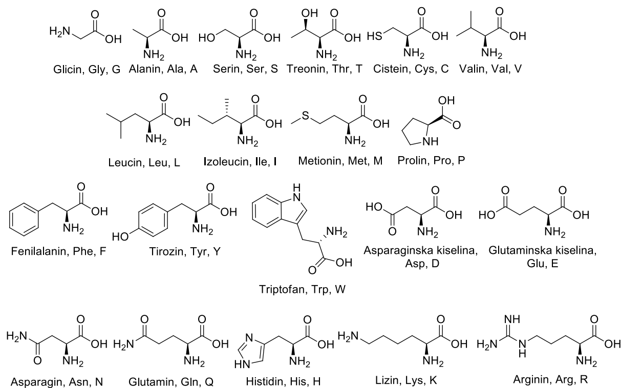
Slika 2. Prikaz strukturnih formula aminokiselina i njihove oznake. 1
