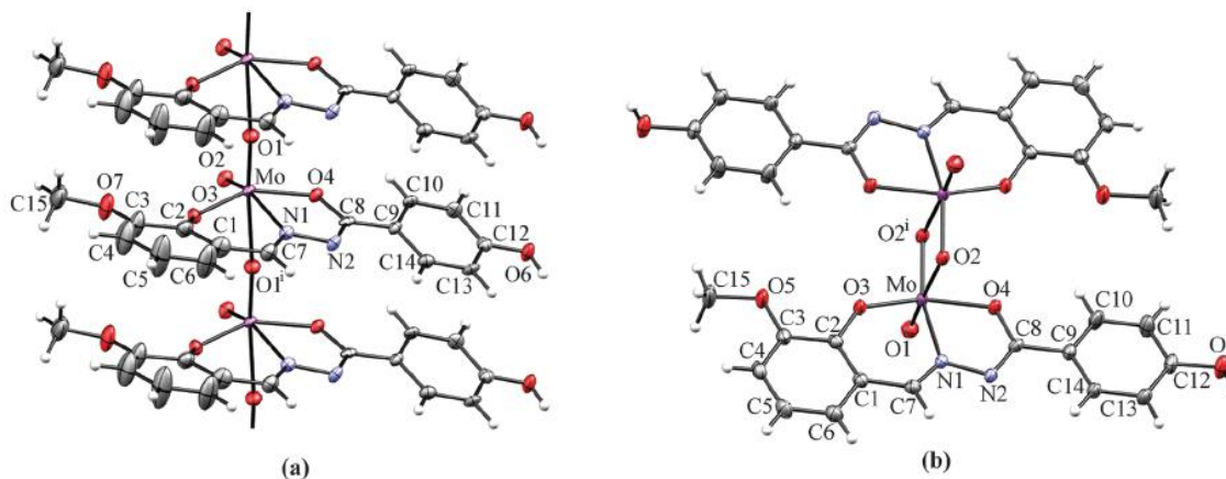
Slika 10. Struktura polinuklearnog kompleksa [\text{MoO}_2(\text{L}^{3\text{OMe}})]_n \cdot \text{MeCN} (a) i dinuklearnog kompleksa [\text{MoO}_2(\text{L}^{3\text{OMe}})]_2 (b). Molekula acetonnitrila je izostavljena radi preglednosti
