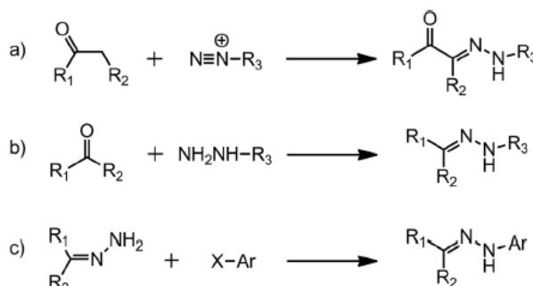
Slika 2. Sintaza hidrazona: a) Japp-Klingemannovom reakcijom, b) reakcijom hidrazina s aldehydom/ketonom, c) supstitucijom aril-halogenida i nesupstituiranih hidrazona
