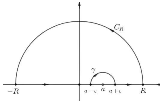
Slika 2.5: Krivulja integracije
