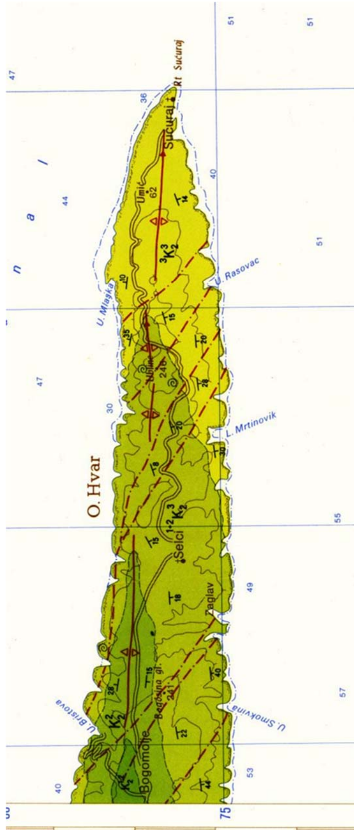
Slika 3. Geološka karta istočnog dijela otoka Hvara. Izvadak iz OGK List Ploče (Marinčić i dr., 1977)
