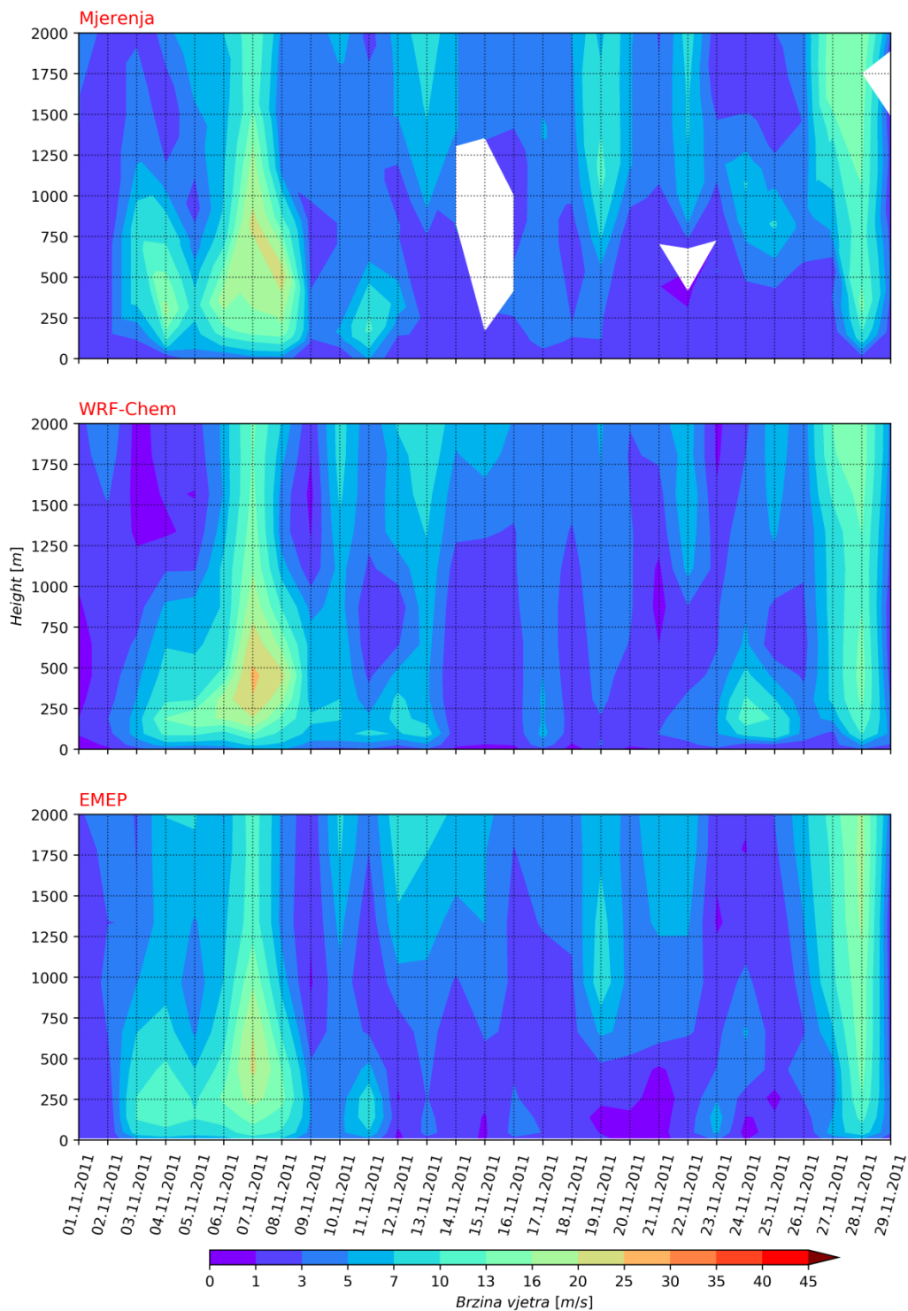
Slika D21. Vremenski niz modeliranog (WRF-Chem i EMEP) i mjenenog vertikalnog profila brzina vjetra na visini do 2000 m za postaju Szeged. Vrijednosti su prikazane za termine u 00 UTC. Nedostatak mjerenih podataka prikazan je bijelom bojom.
