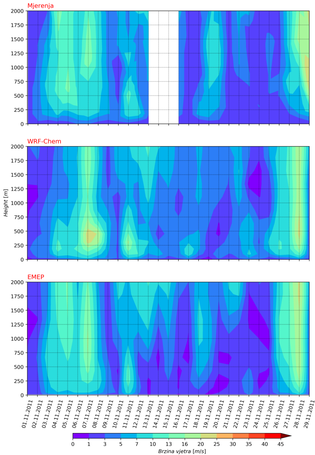
Slika D20. Vremenski niz modeliranog (WRF-Chem i EMEP) i mjenog vertikalnog profila brzina vjetra na visini do 2000 m za postaju Budimpešta. Vrijednosti su prikazane za termine u 00 UTC. Nedostatak mjerenih podataka prikazan je bijelom bojom.
