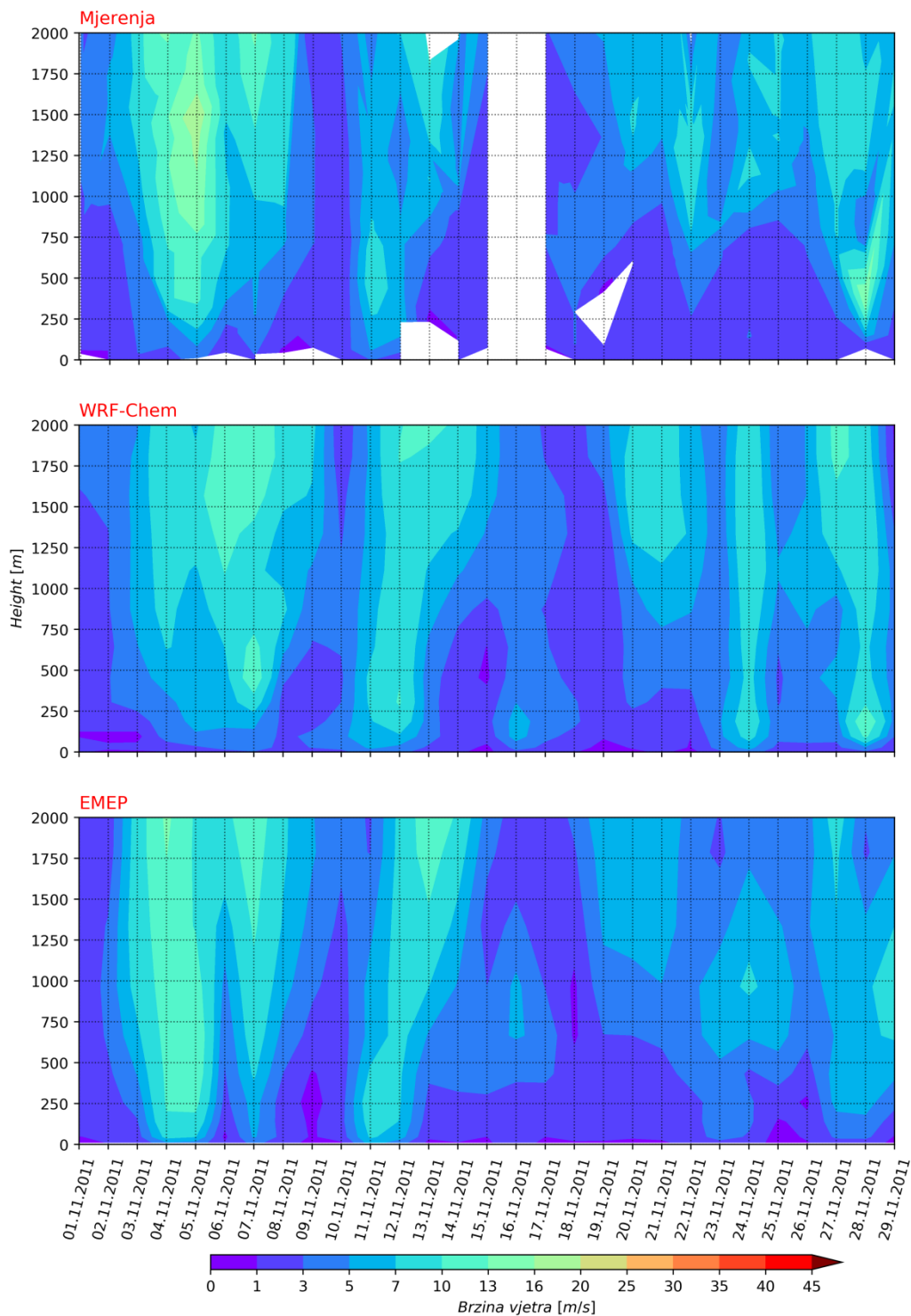
Slika D19. Vremenski niz modeliranog (WRF-Chem i EMEP) i mjenog vertikalnog profila brzina vjetra na visini do 2000 m za lokaciju Zagreb. Vrijednosti su prikazane za termine u 00 UTC. Nedostatak mjenih podataka prikazan je bijelom bojom.
