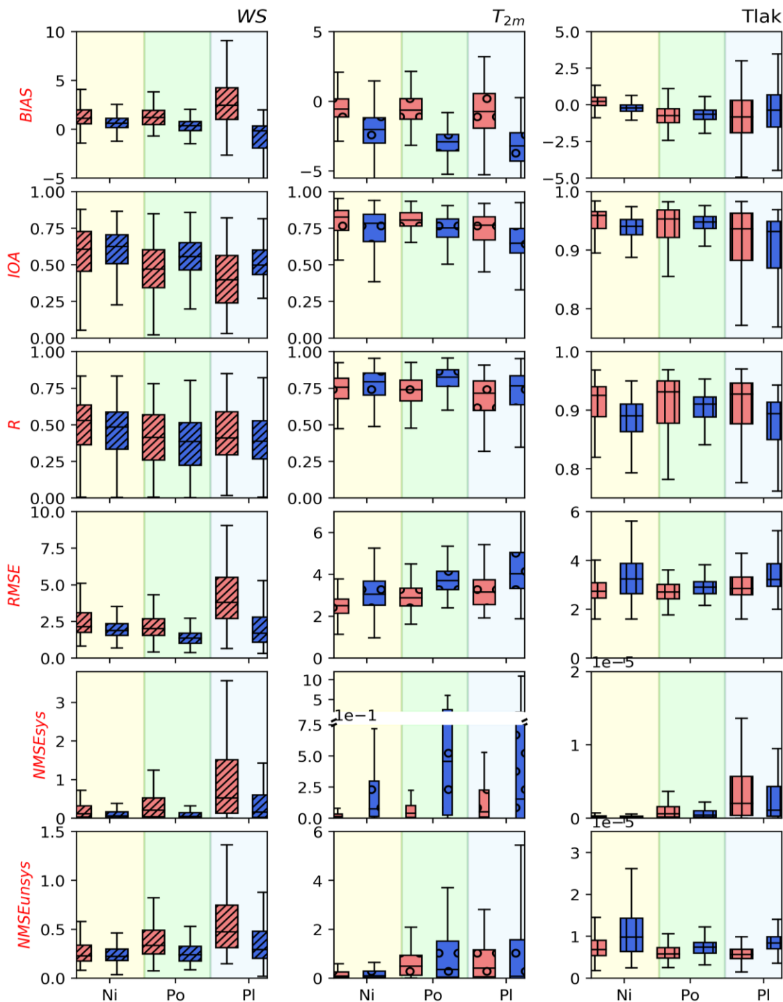
Slika 14. Usporedba statističkih mjera ( BIAS , IOA , r , RMSE , NMSE_{sys} , NMSE_{unsys} ) između modeliranih (WRF-Chem – crveno, EMEP – plavo) i mjerenih (mjerjenja s 920 sinoptičkih postaja diljem Europe) vrijednosti brzine vjetra (WS, //), temperature ( T_{2m} , °) i prizemnog tlaka (Tlak, ||) tijekom studenoga 2011. godine za nizinske postaje (Ni), povišene postaje (Po) te planinske postaje (PI). Mjerne jedinice navedenih parametara su: brzina vjetra [m/s]; temperatura [°C]; prizemni tlak [hPa]. Slika je objavljena u Gašparac i sur. (2020).
