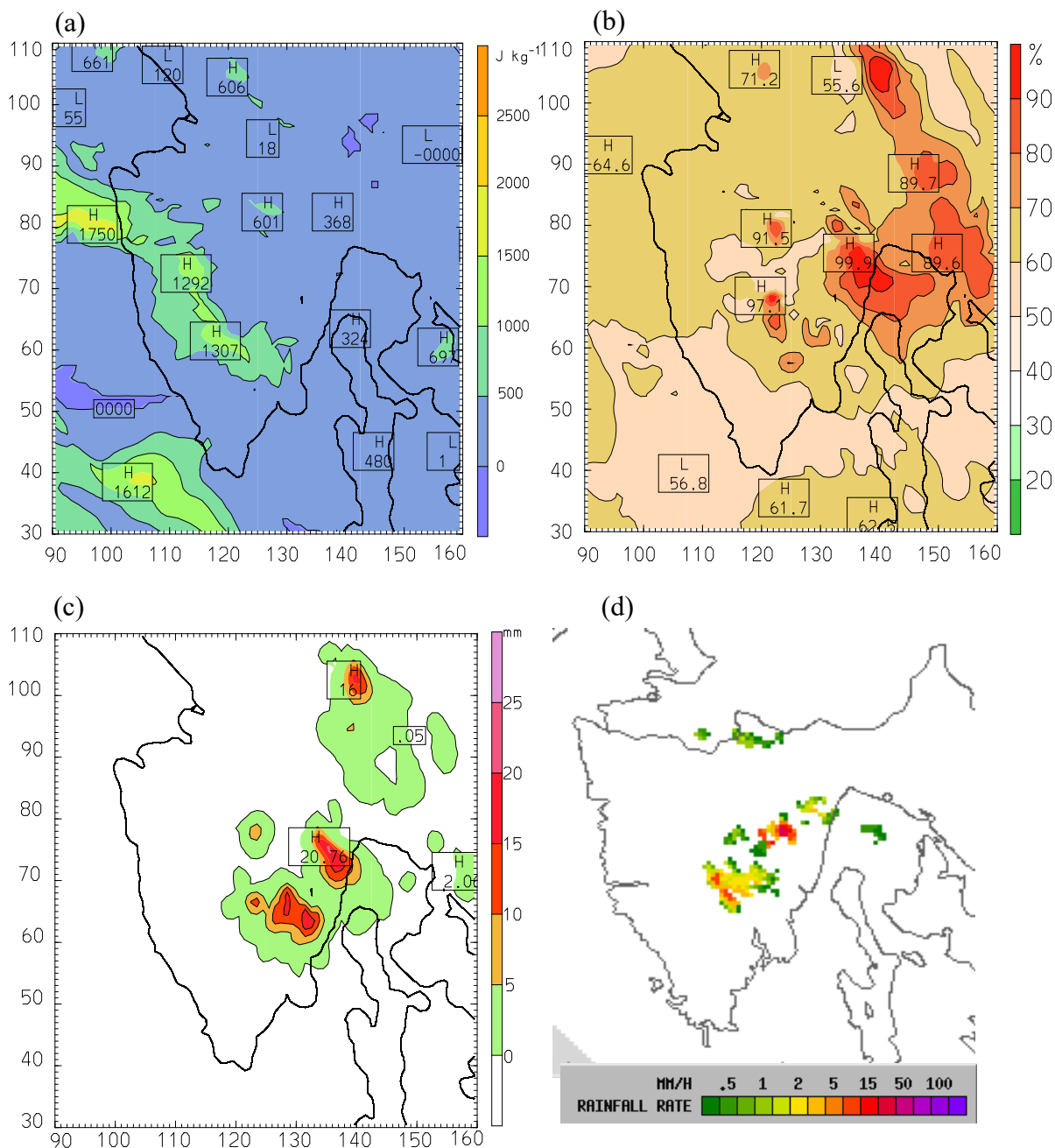
Slika 19: Horizontalna raspodjela (a) CAPE-a ( J kg^{-1} ) u 12:00 CET, (b) usrednjena relativna vlažnost ( rh , %) u sloju između 850 i 500 hPa u 13:00 CET, (c) ukupna količina oborine (mm) dobivena modelom između 13:00 i 14:00 CET, (d) radarska slika maksimalnog intenziteta oborine (mm) u 13:40 CET (izvor: ARSO-www.meteo.si) 8. kolovoza 2006.
