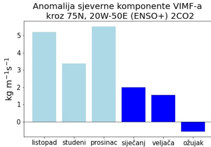
Slika 15. Mjesećne vrijednosti anomalija komponente VIMF-a u smjeru sjever-jug kroz plohu na 20° z.g.d do 50° i.g.d. na 75° s.g.š. za kompozit tople faze ENSO-a (ENSO+) za razdoblje od 1950. do 2010. u toplijoj klimi (2CO2). Svijetloplavo su oznaćeni mjeseci sezone OND za koju je kompozit izraćunat pomoću OND ENSO događaja, a plavom bojom mjeseci JFM izraćunati za JFM ENSO događaje.
