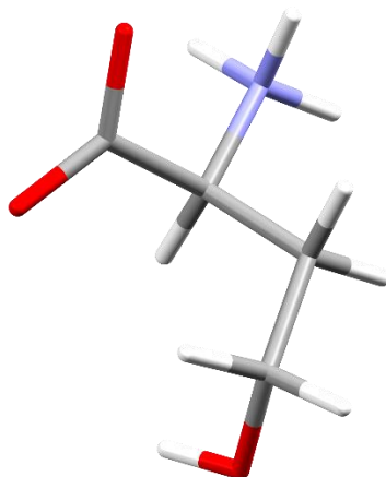
Slika 3. Molekulska struktura L-hososerina, formule C_4H_9NO_3 , kod u CSD bazi BUHG0A01. 34
