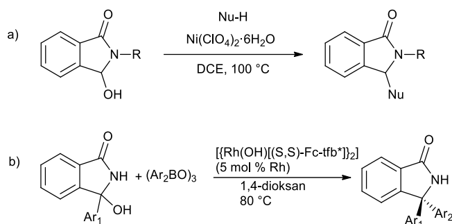
Slika 29. Shematski prikaz: a) nukleofilne supstitucije; b) arilacije 3-amil-3-hidroksiindolinona u prisutnosti Lewisove kiseline
