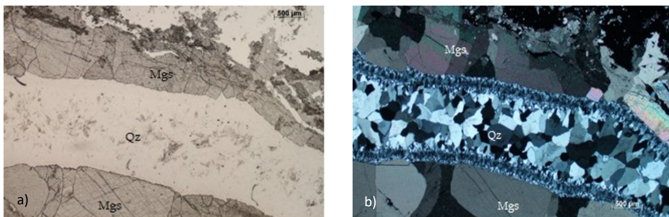
Slika 8. Mikroskopski uzorak Lojane 1 a) bez analizatora b) s analizatorom ( Qz-kremen, Mgs- magnezit); Vidljiva simetrična tekstura
