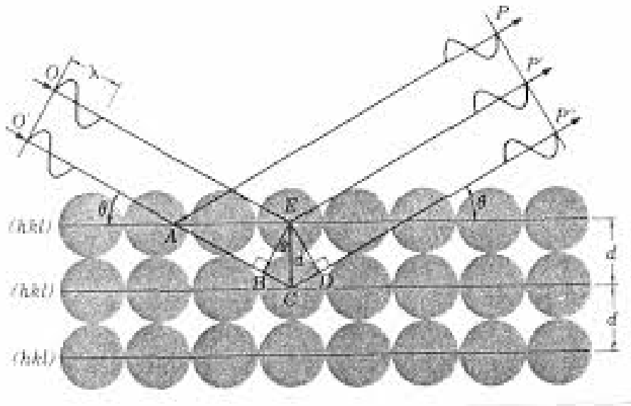
Slika 7. Braggov zakon (Azároff 1968)
