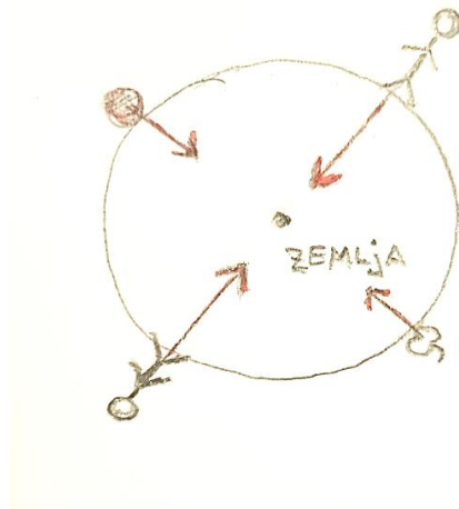
Slika 10 Skica djelovanja gravitacijske sile Zemlje
