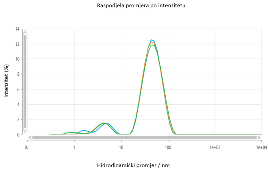
(a) Čisti koloid zlata
