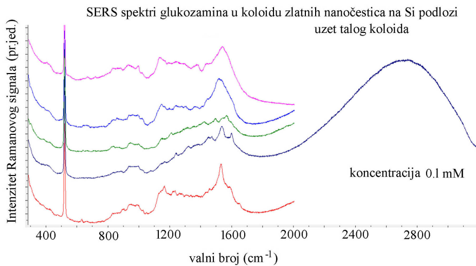
Slika 3.49: SERS spektri glukozamina u koloidu zlata.
