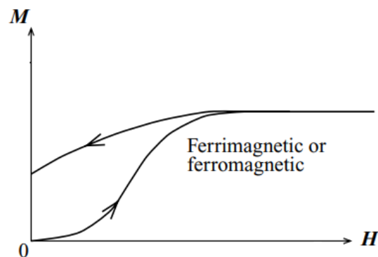
Slika 2.5: Krivulja magnetizacije za feromagnete i ferimagnete [5]
